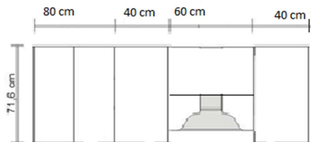
szafka wisząca z pochłaniaczem węglowym
