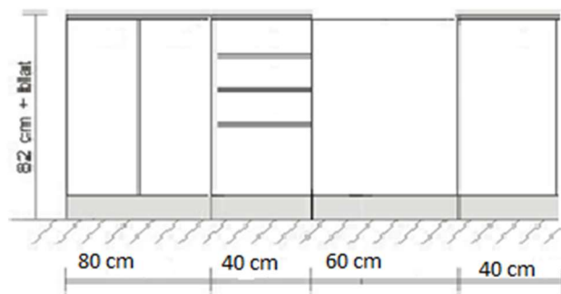
pod zlewozmywak 2 komorowy
